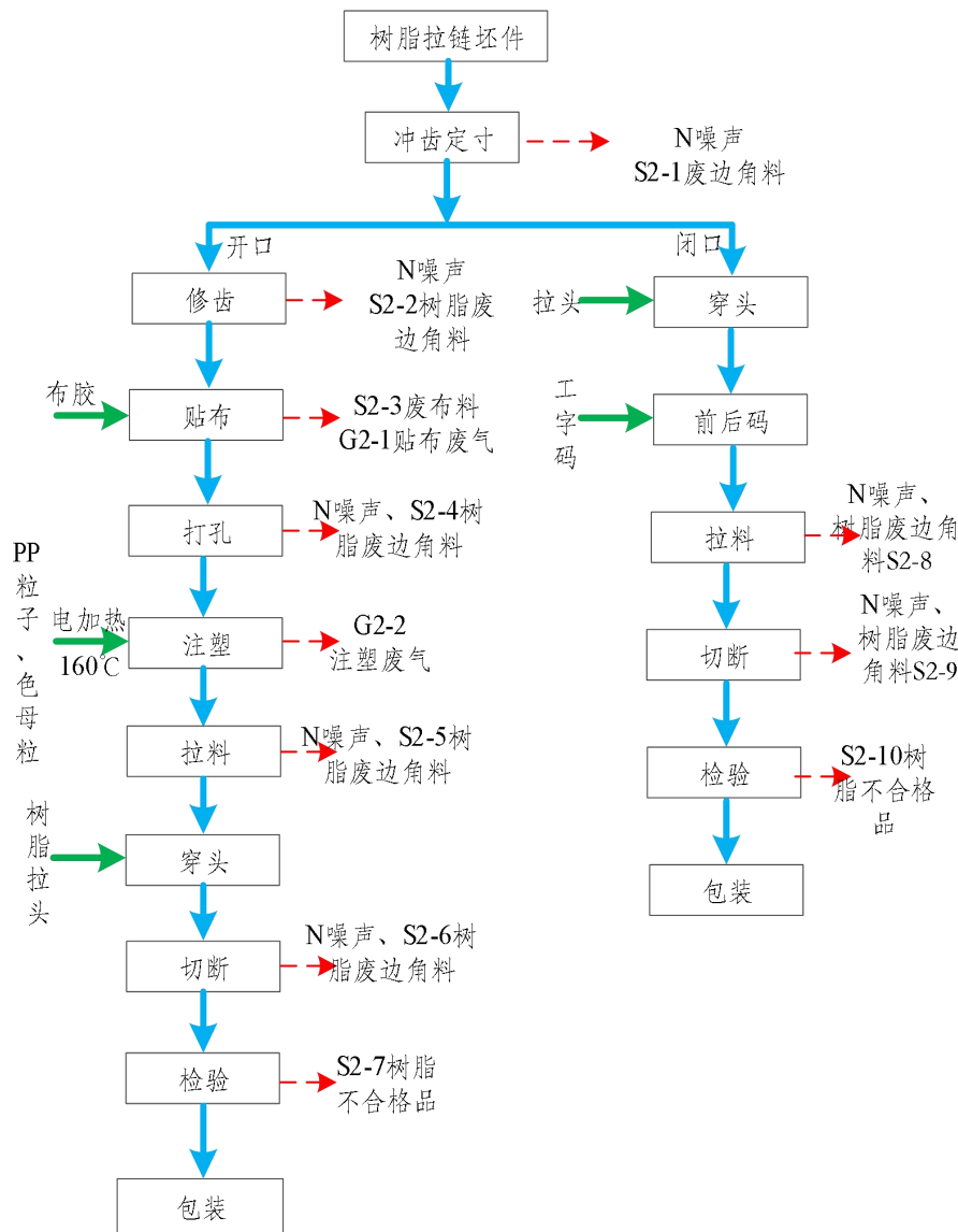
图 2-4 项目树脂拉链加工工艺流程及产污节点图
