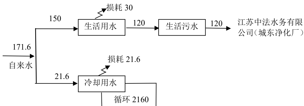
图 2-2 建设项目给排水平衡图单位 t/a
